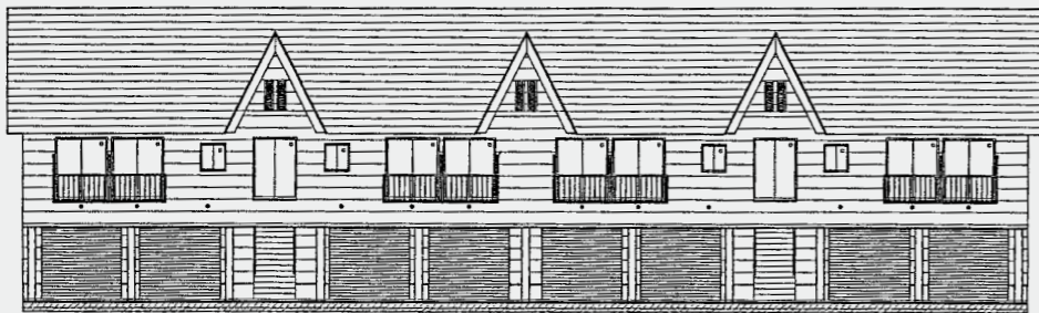
正面立面図
